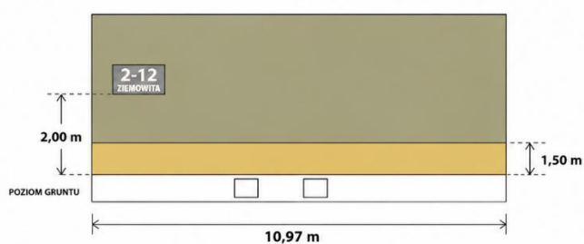
RZUT FRONTOWY (Z WYMIARAMI)
